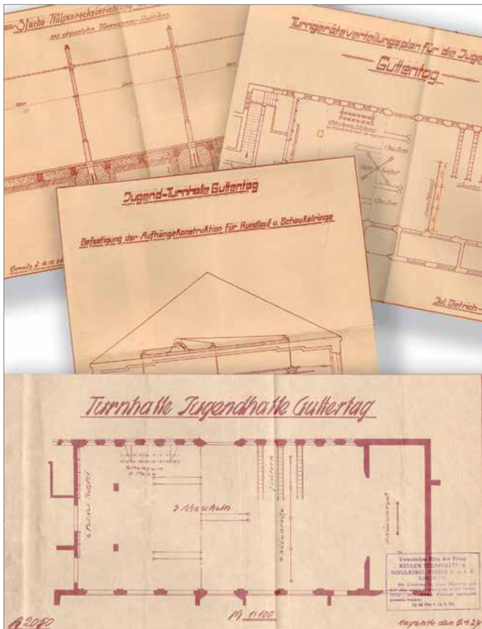
Projekty dotyczące budowy Hali Młodzieżowej w Dobrodzieniu: 1-projekt konstrukcji z zastosowaniem słupów ściennych, wykonanych ze wzmocnionych rur stalowych Mannesmanna (16.12.1926); 2-plan rozmieszczenia sprzętu gimnastycznego w sali sportowej (21.03.1927); 3-projekt mocowania konstrukcji dachu w technologii Polonceau-Binder (21.03.1927); 4-projekt hali sportowej z 5 kwietnia 1927 roku
